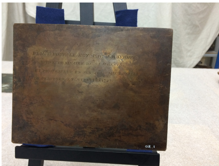
Fig. 2. Support métallique, vue de revers, de Chien en arrêt sur deux faisans (© C2RMF, Johanna Salvant).
